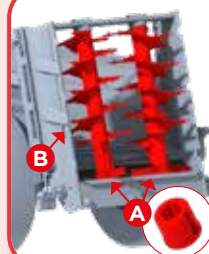
Wałki Ø 820 lub 900 mm zależnie od modelu, zwoje 10 mm.
