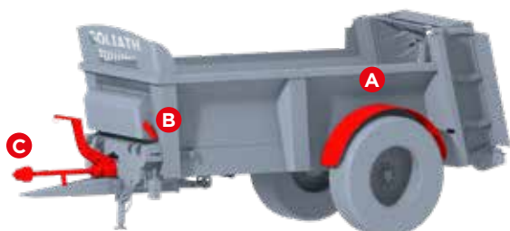
(A) Blotnik stalowy (B) Schówek na dokumenty z indywidualną książką części (C) Uchwyt do przewodów i kardan szerokokątny z zabezpieczeniem krzywkowym.
