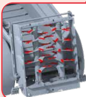
Zęby odwracalne, wymienne ze stali HARDOX 450
