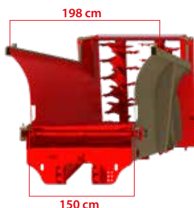
Zaokrąglona skrzynia ułatwiająca rozładunek, wykonana poprzez doginanie blach, by zwiększyć sztywność boków.
